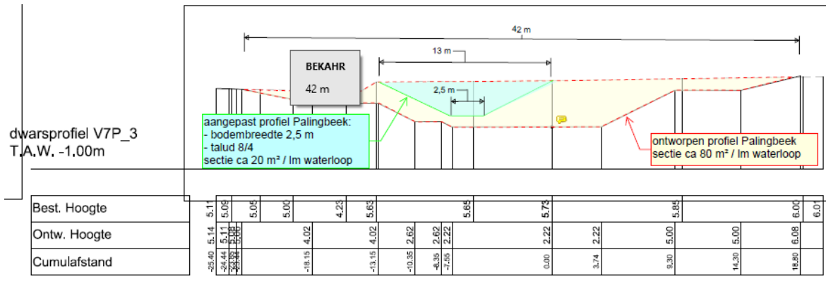
Figuur 3: dwarsprofielen Palingbeek minimaal scenario (blauw) en natuurwaarde scenario (geel) (bron: Lantis)
